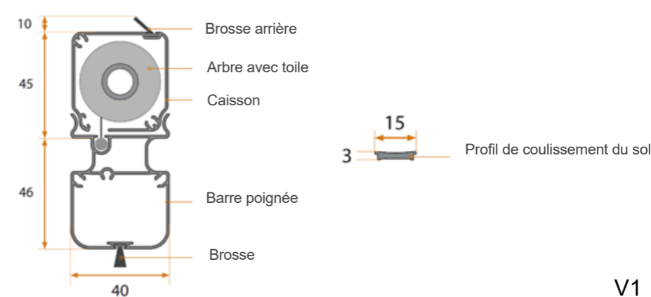
COUPE HORIZONTALE (dimensions en mm)
