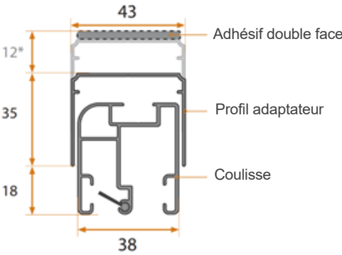
COUPE VERTICALE (dimensions en mm)
