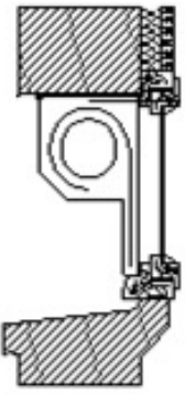
Type de pose n°2 enroulement extérieur
