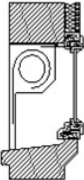
Type de pose n°1 enroulement intérieur
