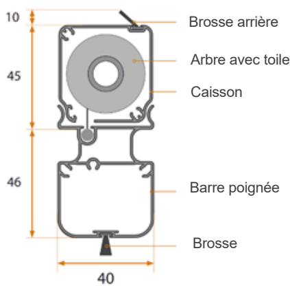
COUPE HORIZONTALE (dimensions en mm)
